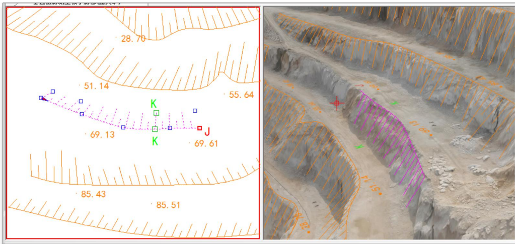
图 6 - 22 斜坡绘制
