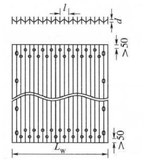
图 8.2.6-5 波纹钢板件拼装 (单位: mm)
