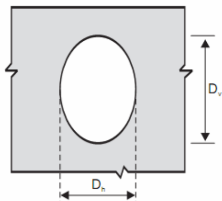
c) 竖向椭圆结构
